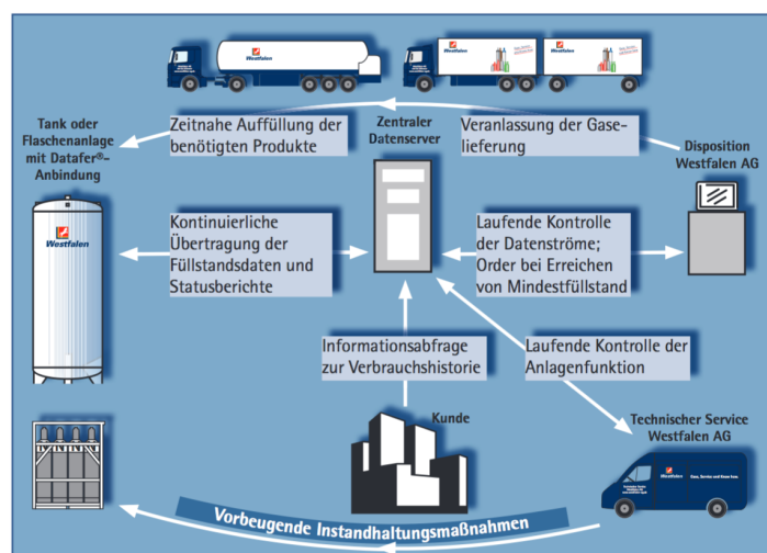
Vereinfachtes Ablaufschema des Datafer®-Systems der Westfalen Gruppe
